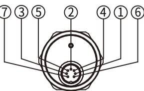
OUTPUT WRP-S-D
