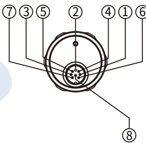
OUTPUT WRP-S-C
